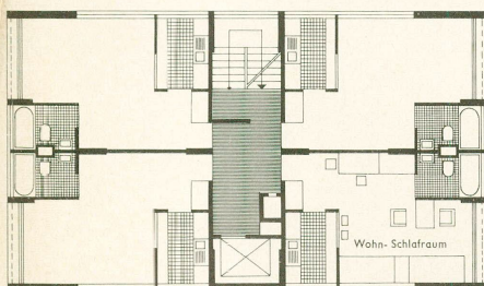
Grundriss, Maßstab 1:200
